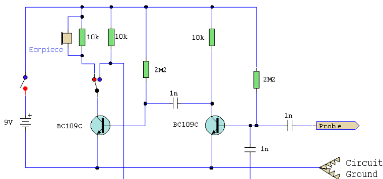
Fig.1 Het schema van de tracer/injector.
