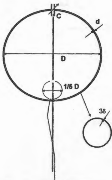
ML met intercontinentale dekking (14-30MHz, D= 75cm).
