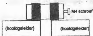
Een hoogspannings-C voor VHF/UHF, gemaakt van coax.
