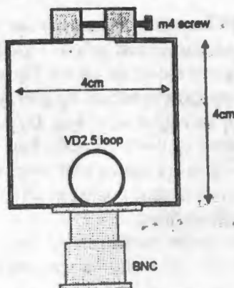
70cm ML, meer dan 6dB beter dan de helix op uw portofoon. In een uurtje zelf te maken.
