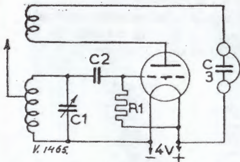
Fig. 2. C_1 = 500 pF, zie tekst; C_2 = 100 pF; C_3 = 1000-3000 pF en R_1 = 1 M \Omega .
